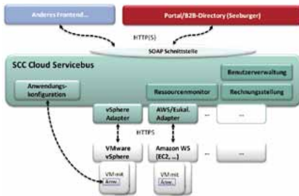
Abbildung 4: SCC Cloud Servicebus (vereinfacht).
