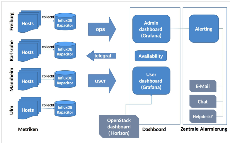
Abb. 3: Architektur der bwCloud-Metrikerfassung – links regional, rechts zentral.
