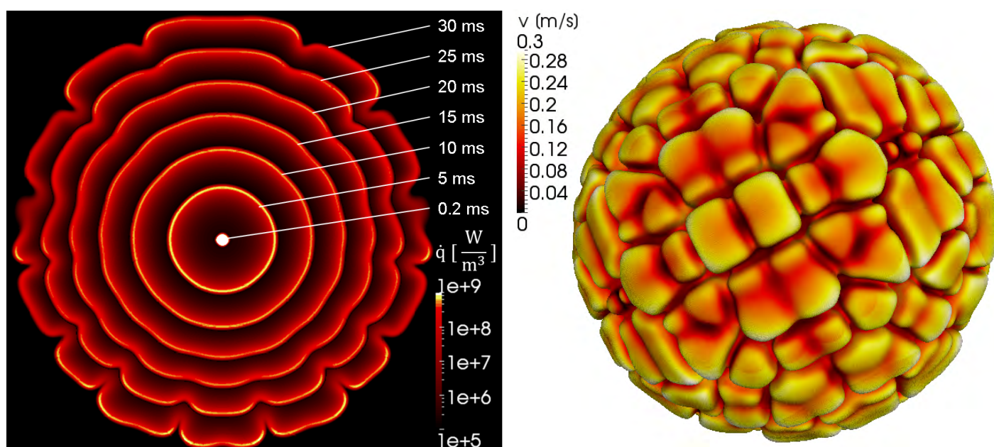
Abb. 1: 3D direkte numerische Simulation der sphärischen Flammenausbreitung: zeitlicher Verlauf der Flammenfront (links) und Snapshot von einer instabilen Flammenoberfläche (rechts).
