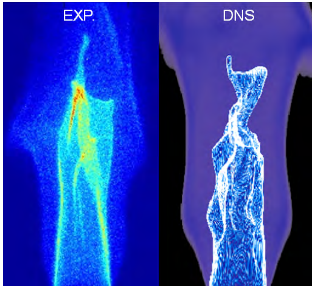
Abb. 2: Vergleich der Chemilumineszenz der Flamme aus der Messung (links) und der Simulation (rechts).
